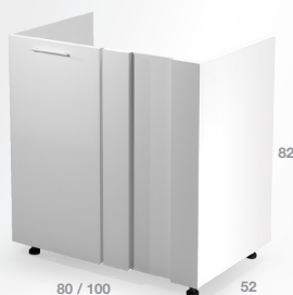
DKN-100(80)/82 sarok mosogató szekrény
