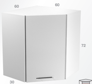
GN-60/72 sarok szekrény
